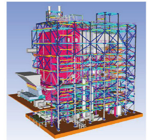
※참조 : 고형연료 열공급시설 건설공사 적용 Combustion & Boiler Package
